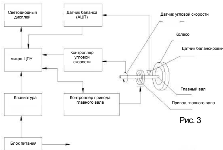
Рис. 3 Функциональная блок-схема балансировочного станка СВ1930Е
